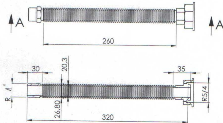
presek A-A
